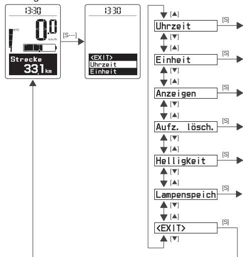
Hauptfahran- zeige
